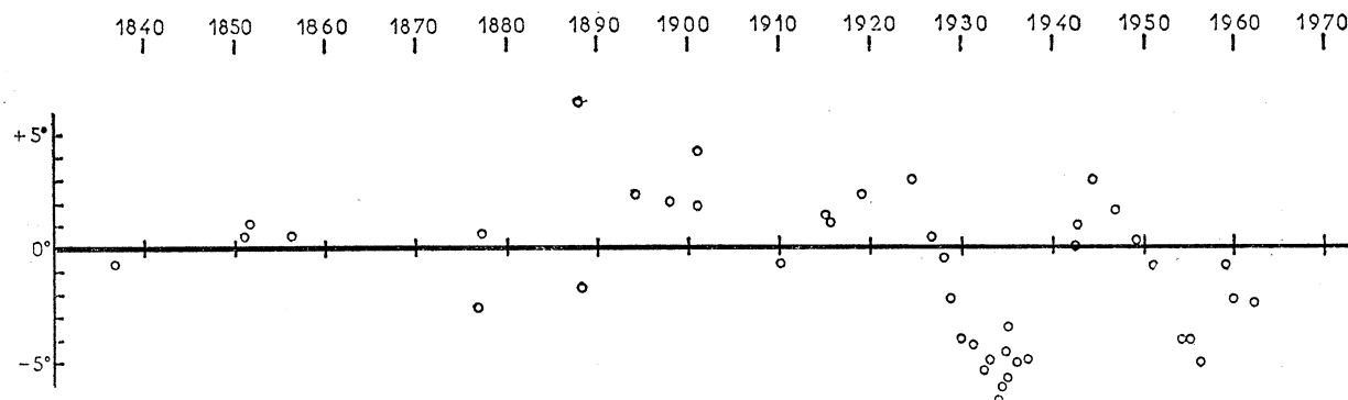
FIG. 2. Les résidus O - C pour le système AC.
