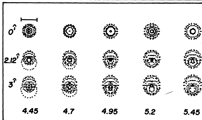
Diagrama 5. interferómetro fabry-perot (f/13.5) campo utilizado: 6 min. arc. corrimiento de foco: 4.95 inc.: 0.25mm.
