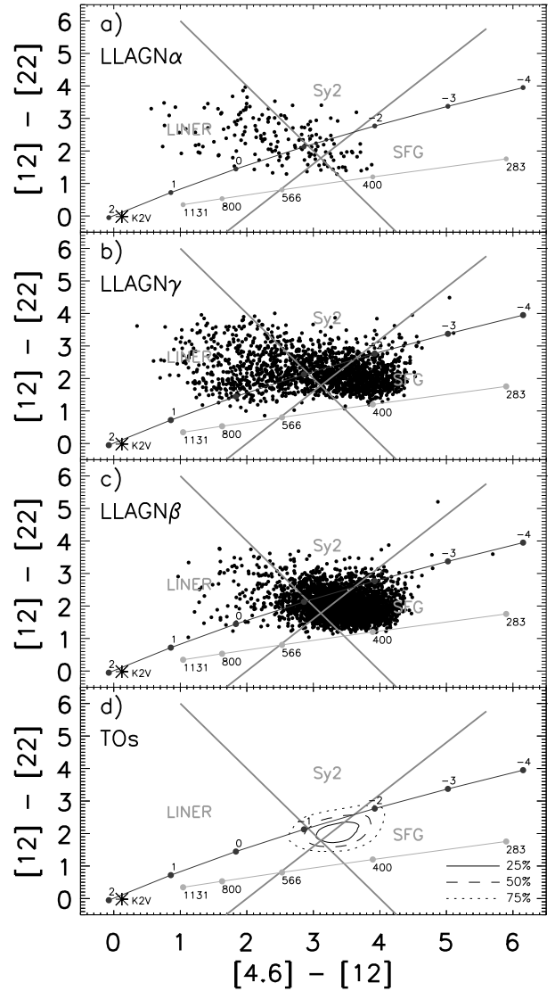
Fig. 15. The MIR diagnostic diagram for a) the LLAGN \alpha , b) the LLAGN \gamma , c) the LLAGN \beta , and d) the TOs.
